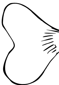
queue
